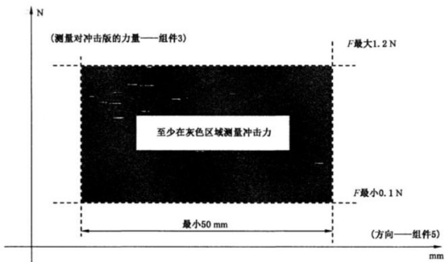
图 11 冲击力分布
